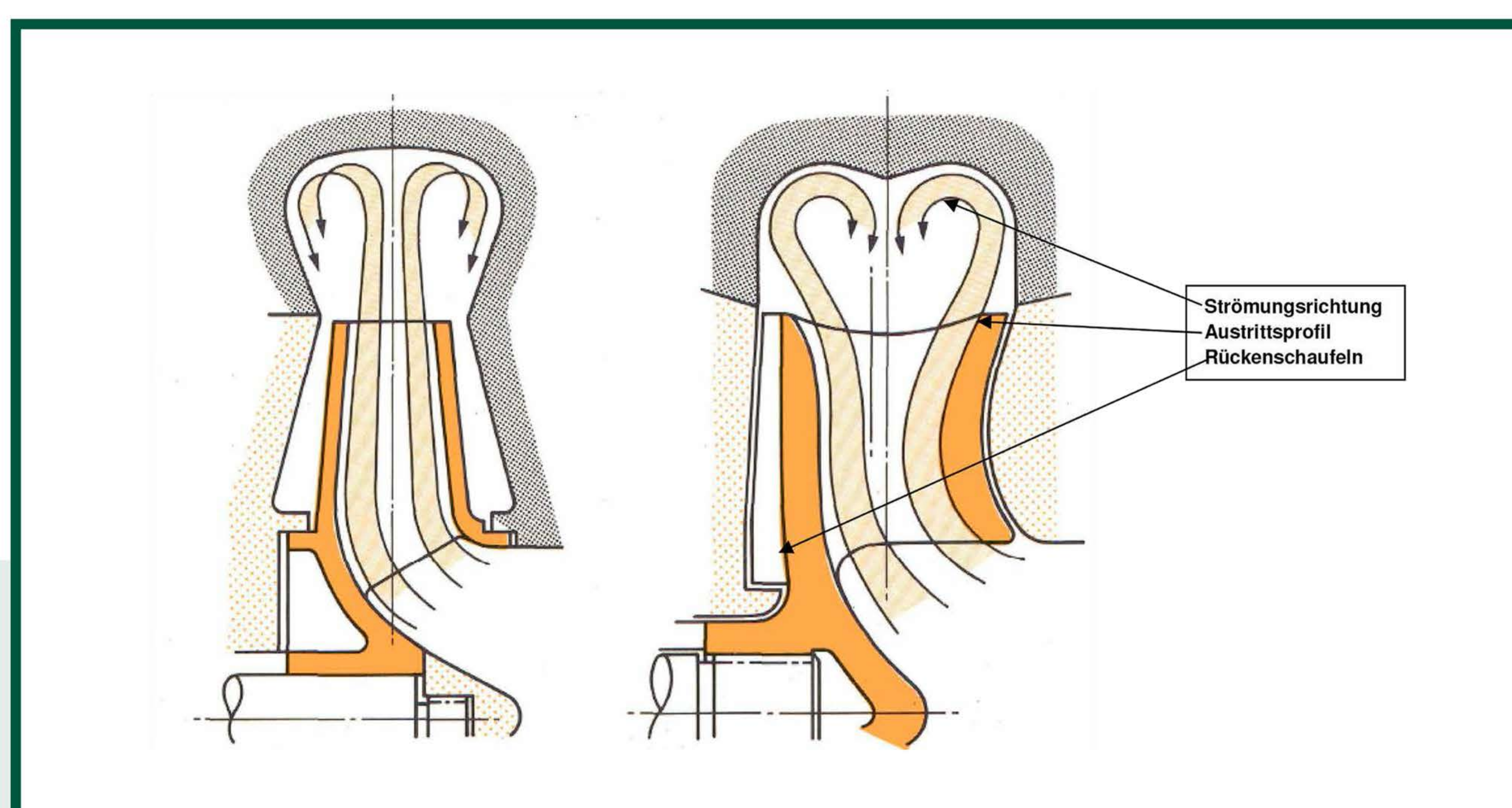
Конструкция рабочего колеса Glass & Wolff Lauftradkonstruktion Glass & Wolff impeller design Glass & Wolff
