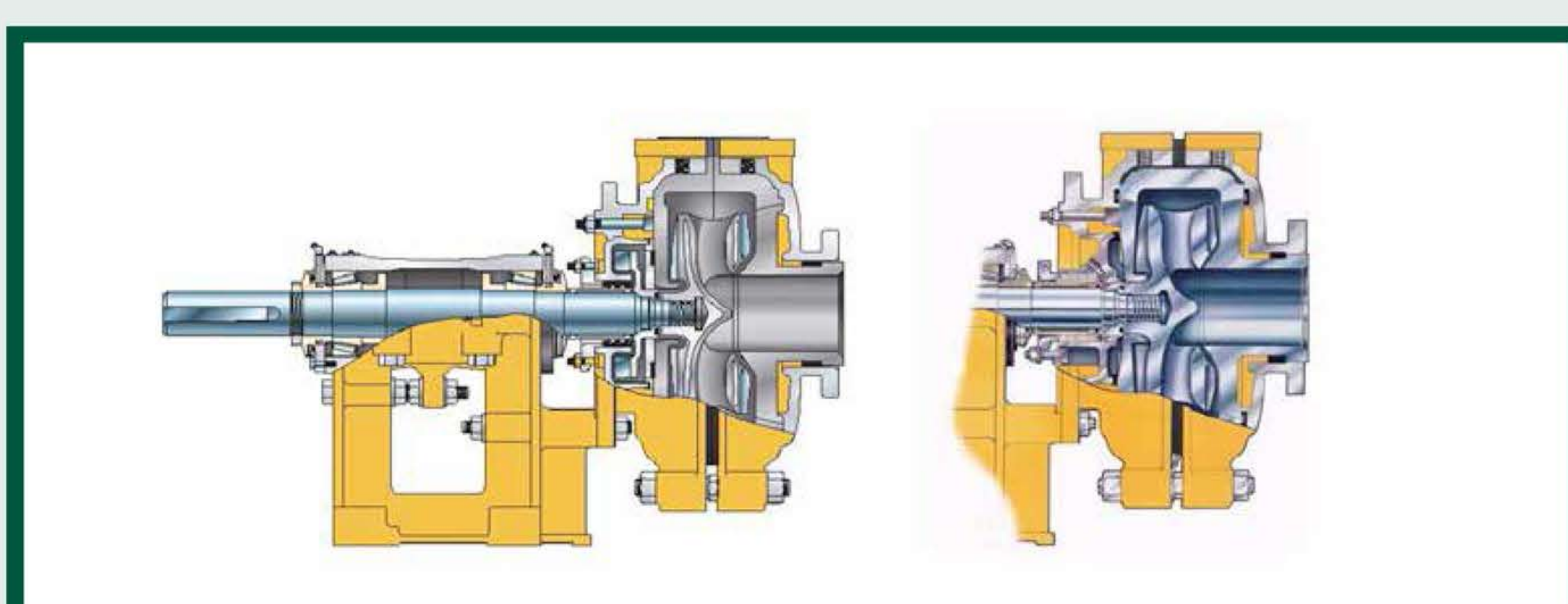
Разрез насоса Pumpeschnitt pump section
